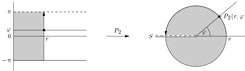
Abbildung des Streifens \mathbb{R}_+ \times (-\pi; \pi) auf die geschlitzte Ebene \mathbb{R}^2 \setminus S
