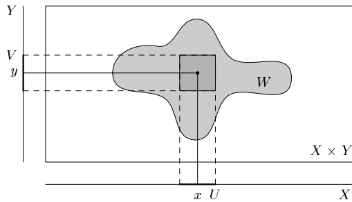
Definition der Produkttopologie
