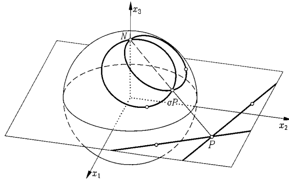
Abbildung zweier Geraden durch stereographische Projektion
